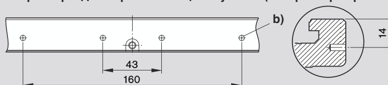
b) M4 - 6 глб.
