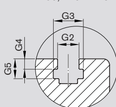
Вид А Типоразмер каркаса 90, 110 и 145
