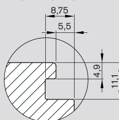
Вид А Типоразмер каркаса 200
