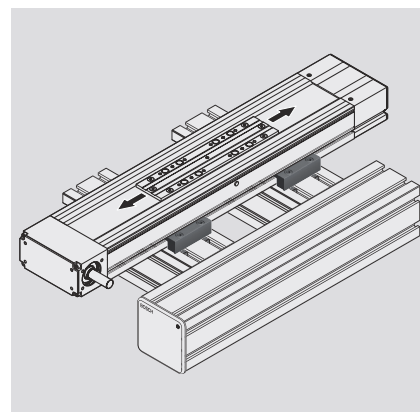
Соединительные элементы для крепления компактных модулей
