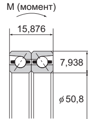
Радиально-упорный подшипник
