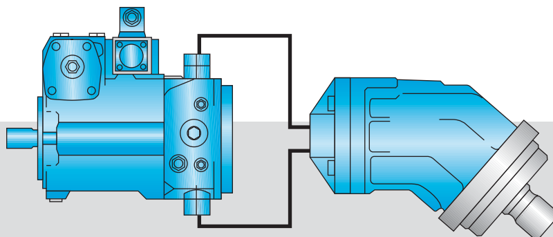
Гидростатический привод A10VG/ A2FM
