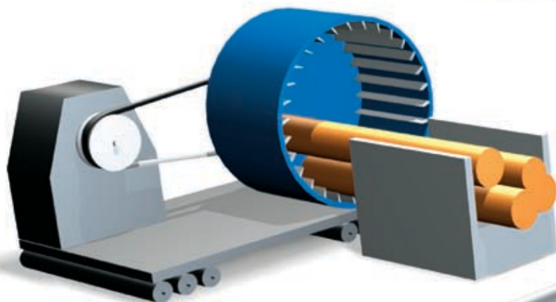
Тиски для ножевого роторного стружечного станка
