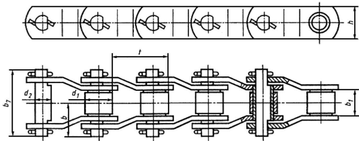
Рисунок 7 - Цепь типа ПРИ
