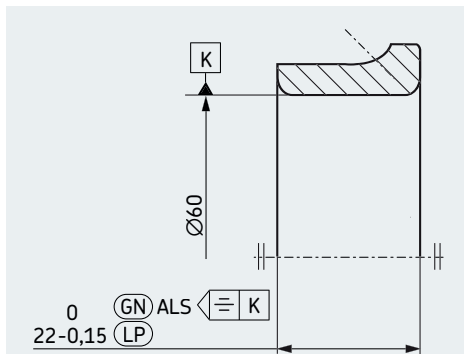
Рис. 4: Пример указания допуска ширины внутреннего кольца радиально-упорного шарикоподшипника.
